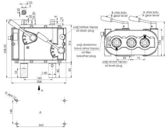
DİŞLİ DÜZENİ / GEAR ARRANGEMENT
