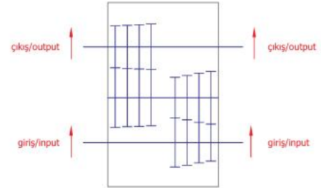
DİŞLİ DÜZENİ / GEAR ARRANGEMENT
